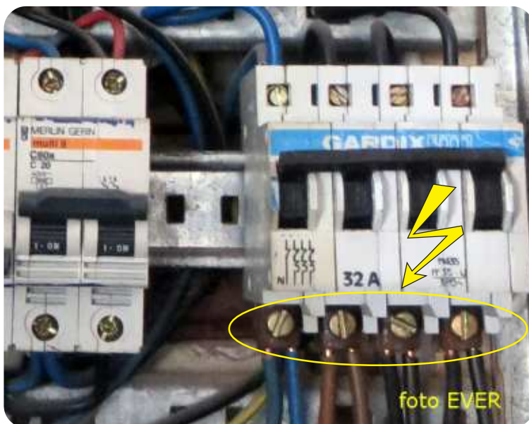
Rechts : Hoofdschakelaar is een automaat van 32A 3kA
