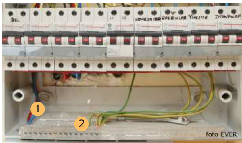
Voeding van het ALSB met VOB draden -1- onaanvaardbaar, sectie duidelijk ondermaats en doorvoer strijdig met artikel 201-205 AREI. De beschermingsgeleiders van de ganse elektrische installatie -2- zijn niet aangesloten op een aarding, art. 69-71 van het AREI.
