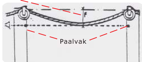
Voorstelling van de "doorhang / pijl" van de kabel waarbij de trekkracht wordt bepaald.
