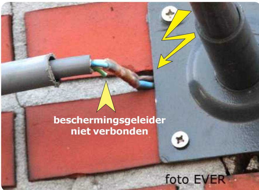
Tremelo : aansluiting gevelverlichting Cadeau-factory
