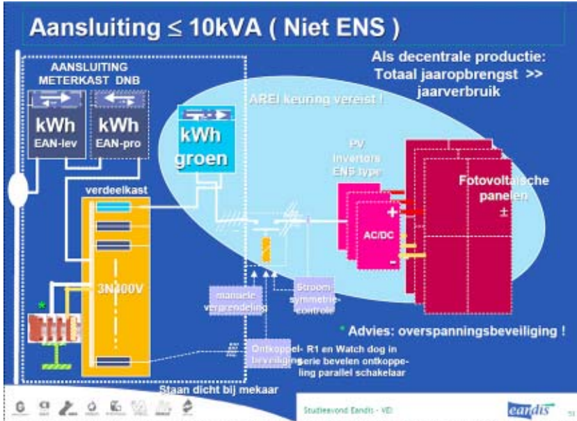
Zo zal een 2-weg aansluiting (niet ENS -zonder ontkoppelrelais), er uitzien, wat denkt ge wie dat allemaal gaat betalen ? - Slide EANDIS.
