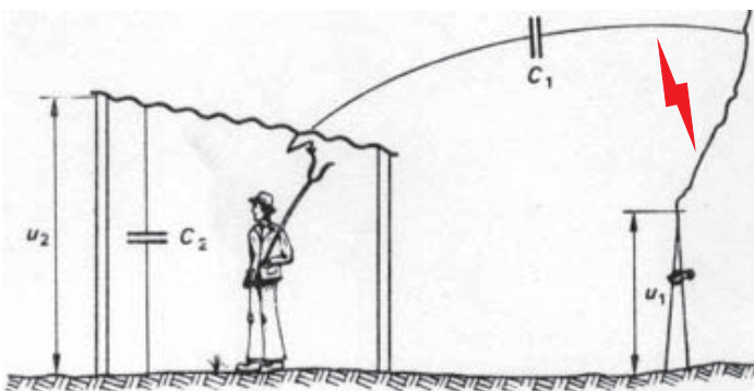
Voorstelling uit de cursus van de Faculté Polytechnique de Mons van een inductieverschijnsel op een metalen dak.
